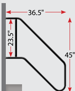
AC-544L
